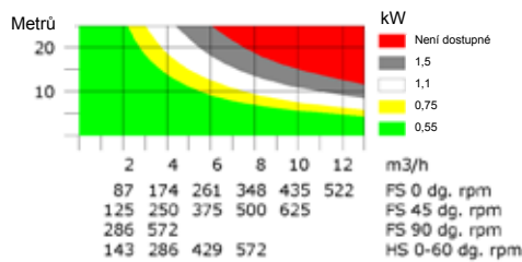
Výkonnosti dopravníků Ø102 mm
