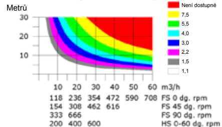
Výkonnosti dopravníků Ø152 mm
